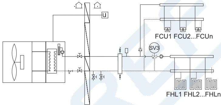
uspořádání systému 3
