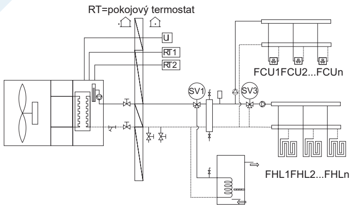
uspořádání systému 4
